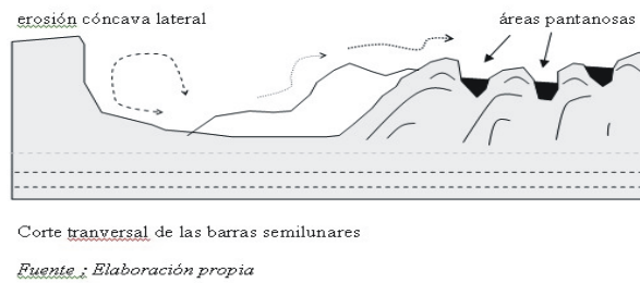
Figura 17. Corte transversal de las barras semilunares. Elaboración propia
