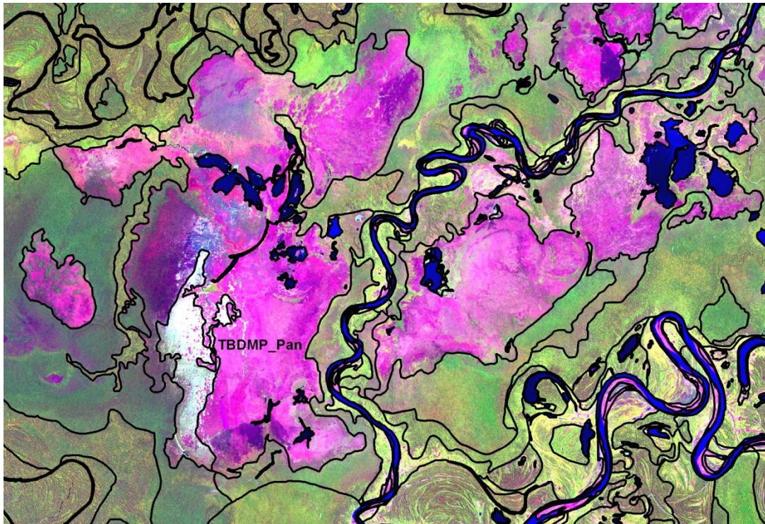
Figura 20. Relieve de cubeta fluviopalustre, el cual se encuentra colmatado por sedimentos orgánicos, conformando vegetación de tipo "pantano". Reserva Nacional Pacaya Samiria. Imagen Landsat 2008.
